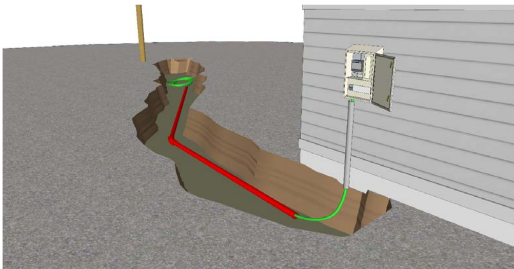
Figur 3 RT11069 Jordkabel fra stolpe
